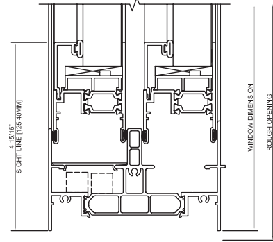
405 JAMB
