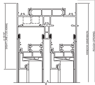
401 JAMB
